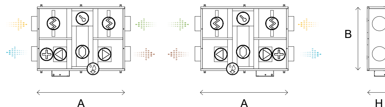
WIDOK Z GÓRY (przeciwny do strony obsługowej) WERSJA LEWA TOP VIEW (opposite to the operating site) LEFT VERSION
