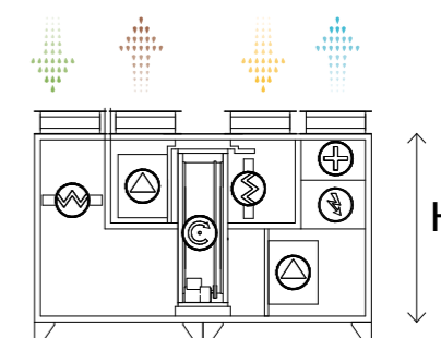
WIDOK OD STRONY OBSŁUGOWEJ WERSJA PRAWA
