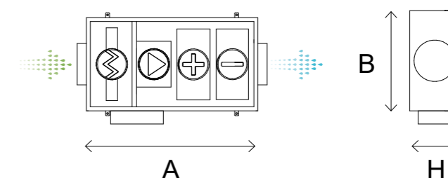
WIDOK Z GÓRY (przeciwny do strony obsługowej) WERSJA PRAWA TOP VIEW (opposite to the operating site) RIGHT VERSION
