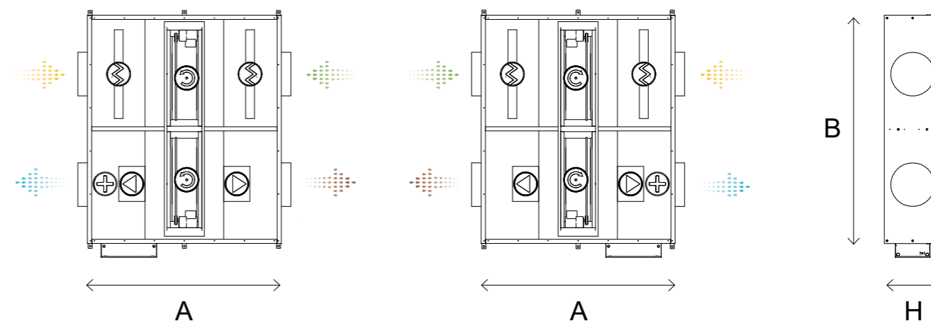
WIDOK Z GÓRY (przeciwny do strony obsługowej) WERSJA LEWA
