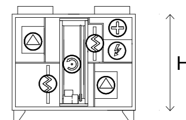
WIDOK OD STRONY OBSŁUGOWEJ WERSJA PRAWA
