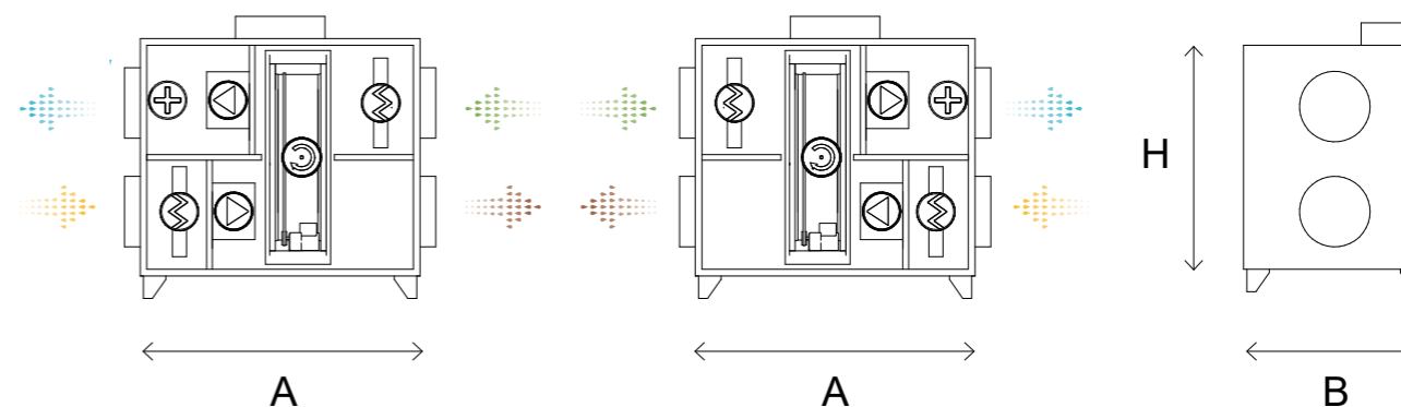
WIDOK OD STRONY OBSŁUGOWEJ WERSJA LEWA
