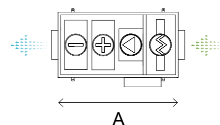
WIDOK Z GÓRY (przeciwny do strony obsługowej) WERSJA LEWA TOP VIEW (opposite to the operating site) LEFT VERSION
