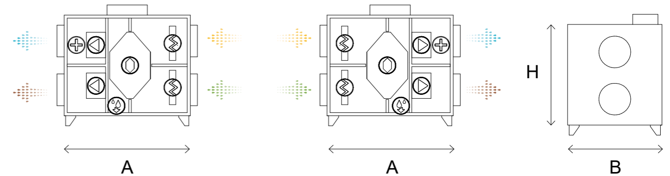
WIDOK OD STRONY OBSŁUGOWEJ WERSJA LEWA
